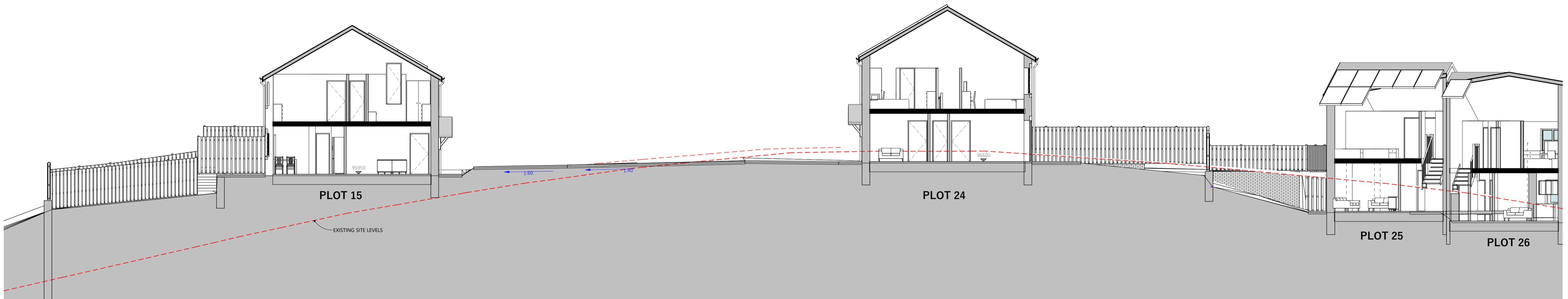
SECTION E-E SCALE: 1 : 100
