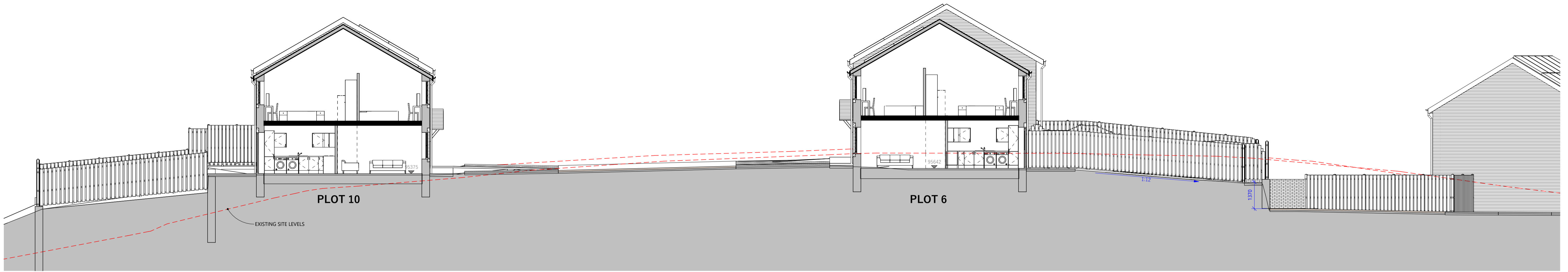
SECTION D-D SCALE: 1 : 100
