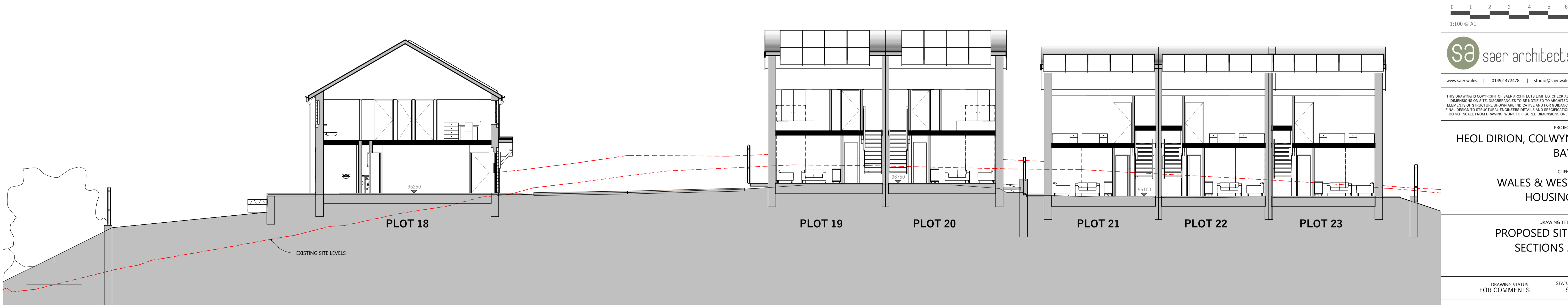
SECTION F-F SCALE: 1 : 100
