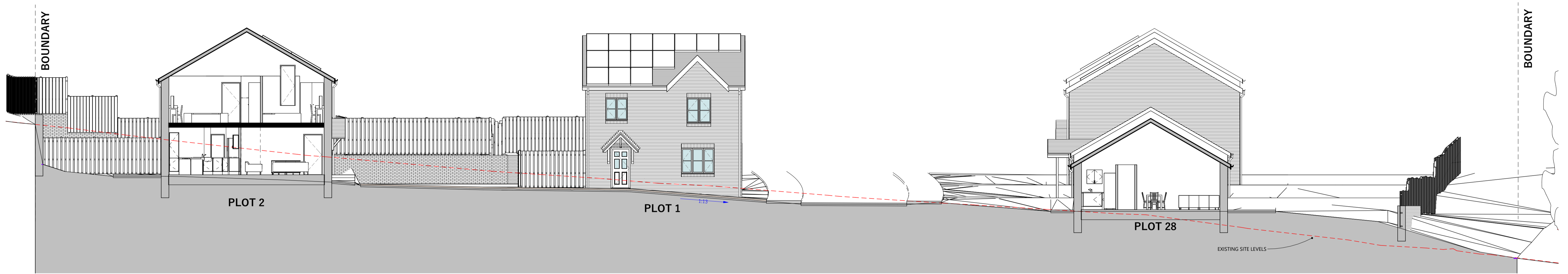
SECTION H-H SCALE: 1:100
